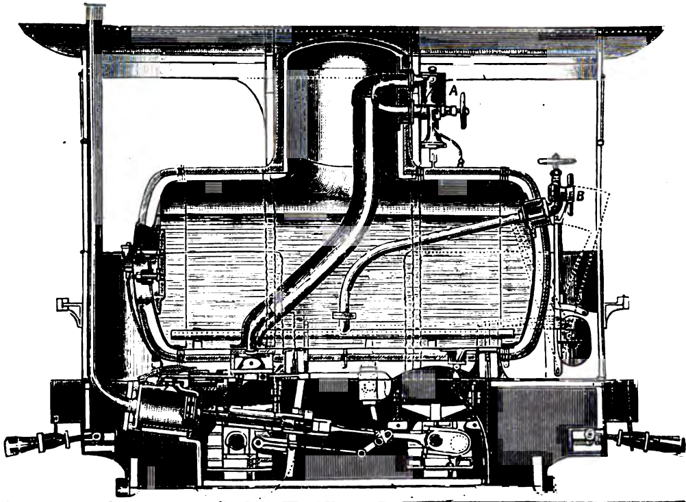
1. Локомотивъ Ламъ Франка (разрѣзъ).
